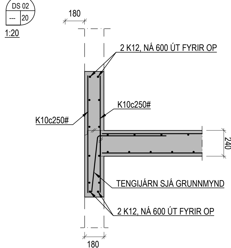
DÆMIGERT SNIÐ: TENING MILLIPLÖTU VIÐ ÚTVEGGI ÞAR SEM GLUGGAR ERU FYRIR OFAN OG NEÐAN PLÖTU 1:20
