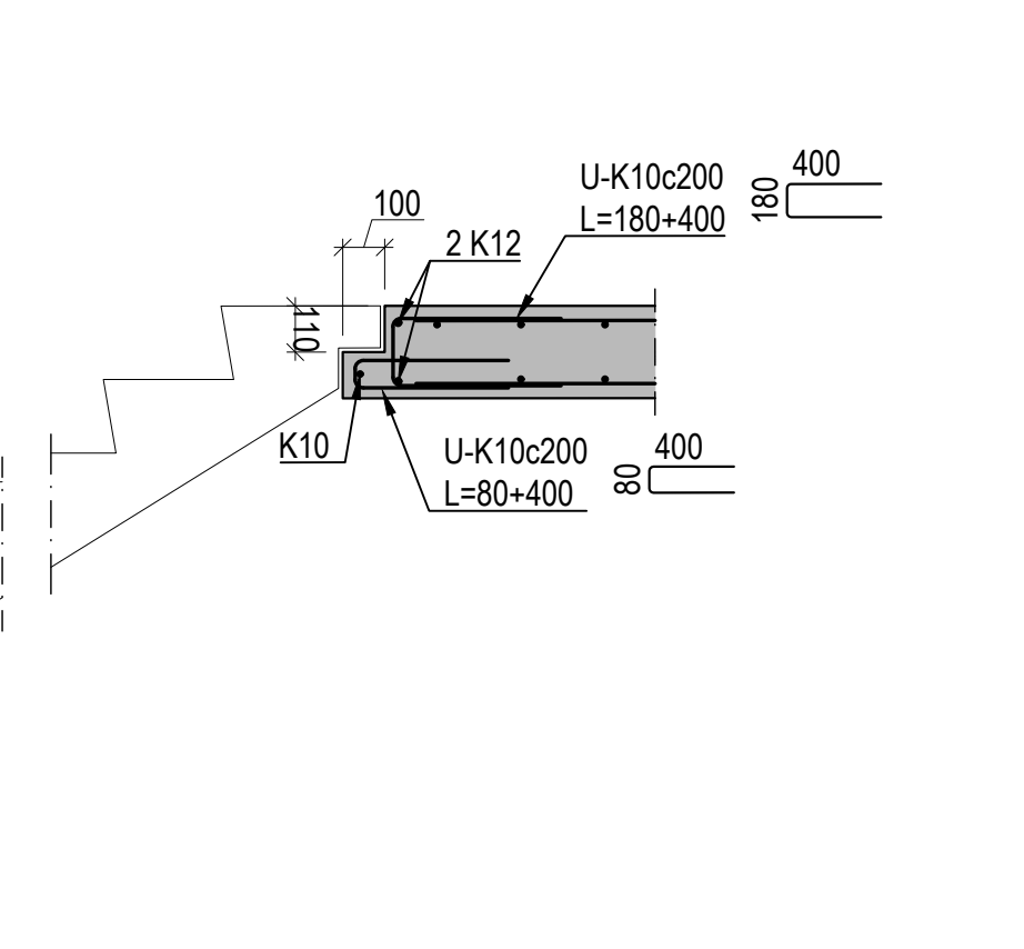
DÆMIGERT SNIÐ: TENING PLÖTU VIÐ INNVEGGI 1:20
