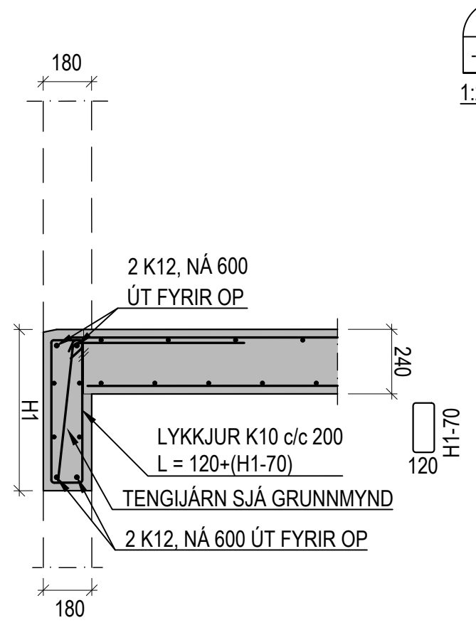
DÆMIGERT SNIÐ: TENING MILLIPLÖTU VIÐ ÚTVEGGI ÞAR SEM HURÐIR / GÖLFSÍÐIR GLUGGAR ERU FYRIR OFAN OG NEÐAN PLÖTU 1:20
