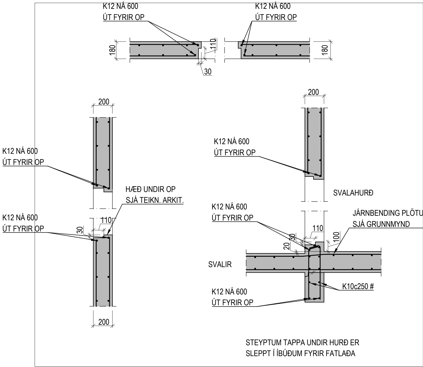
DÆMIGERÐ SNIÐ VIÐ GLUGGA OG HURÐIR
