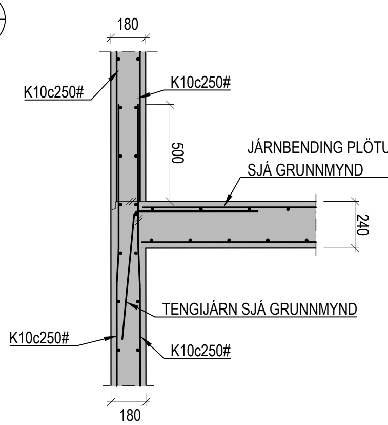
DÆMIGERT SNIÐ: TENING MILLIPLÖTU VIÐ ÚTVEGGI 1:20
