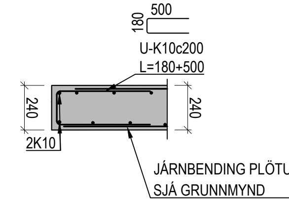
DÆMIGERT SNIÐ: VEGGENDI VIÐ LYFTUHURÐIR
