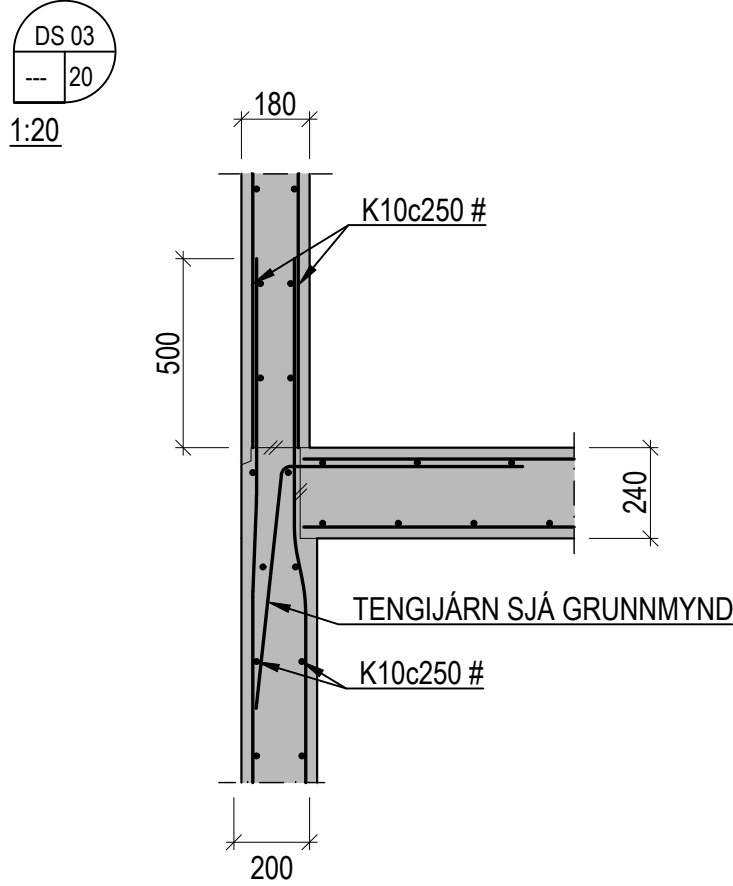
DÆMIGERT SNIÐ: TENING MILLIPLÖTU VIÐ ÚTVEGGI Þ.S. ÚTVEGGUR MJÓKKAR ÚR 200 Í 180 MM
