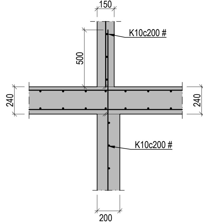
DÆMIGERT SNIÐ: TENING PLÖTU VIÐ INNVEGGI Þ.S. INNVEGGUR MJÓKKAR ÚR 200 Í 150 MM
