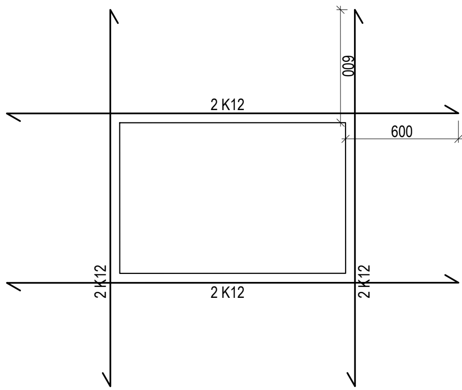
DÆMIGERT SNIÐ: JÄRNBENDING Í KRINGUM GLUGGA OG HURÐIR 1:20
