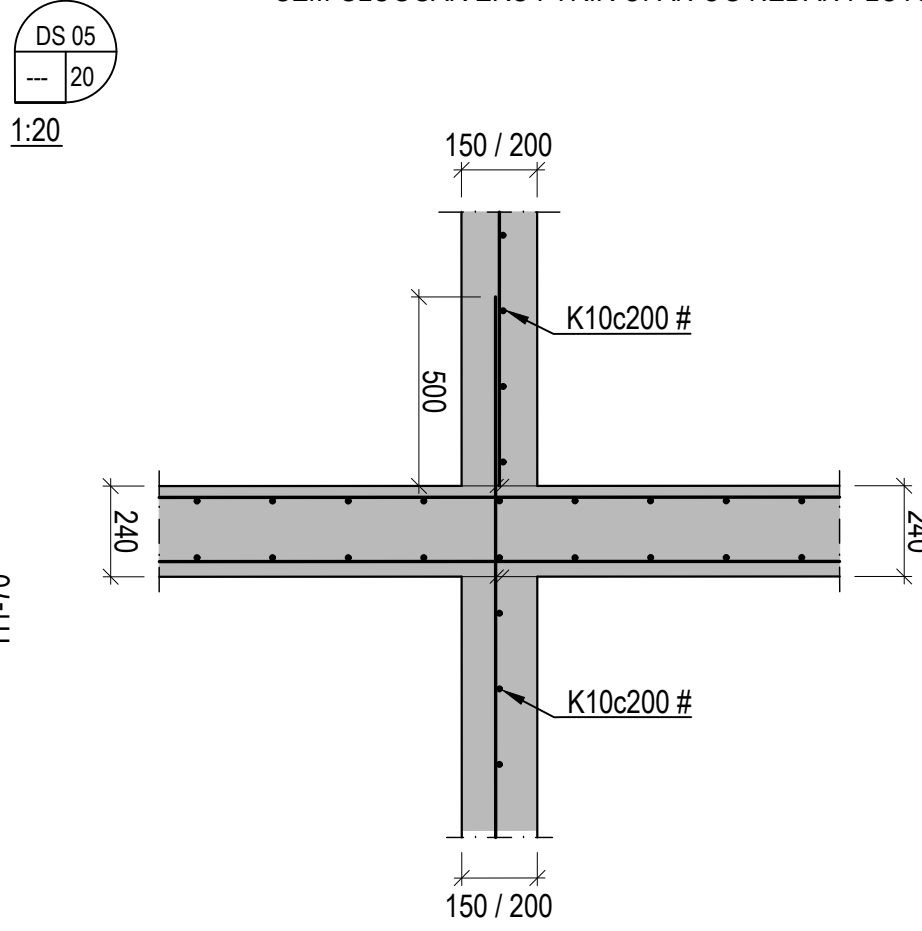
DÆMIGERT SNIÐ: TENING PLÖTU VIÐ INNVEGGI 1:20
