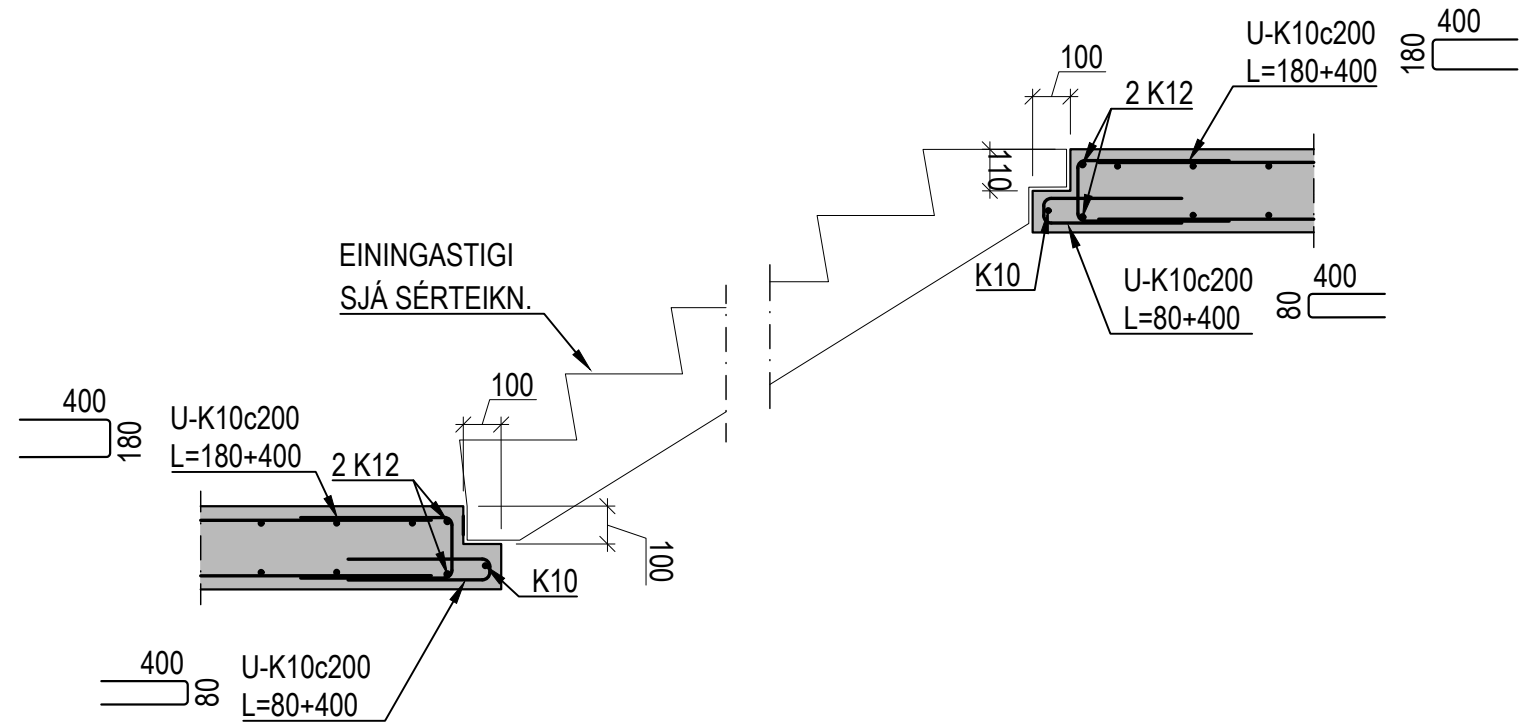
DÆMIGERT SNIÐ: SÆTI FYRIR EININGASTIGA
