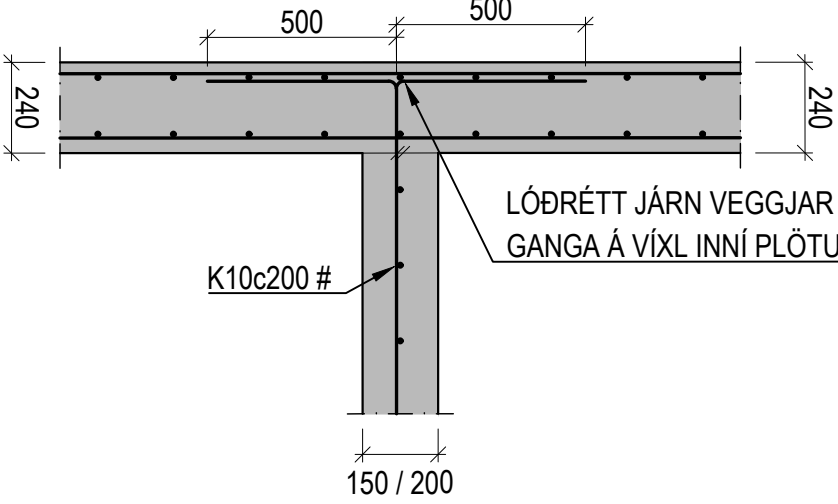
DÆMIGERT SNIÐ: TENING PLÖTU VIÐ INNVEGGI ÞAR SEM EKKI ER VEGGUR FYRIR OFAN PLÖTU 1:20
