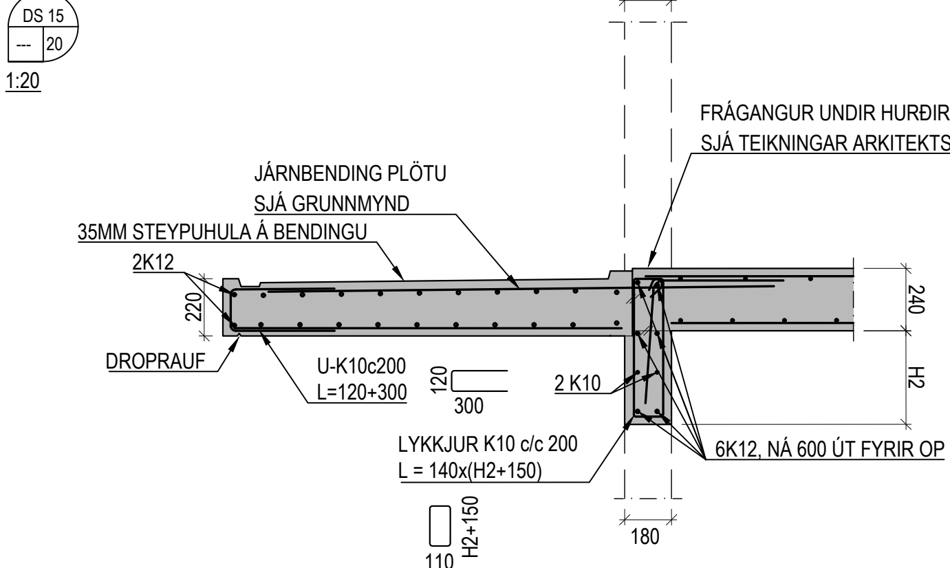
DÆMIGERT SNIÐ: TENING MILLIPLÖTU VIÐ ÚTVEGGI VIÐ SVALAHURÐIR / GÖLFSÍÐA GLUGGA 1:20
