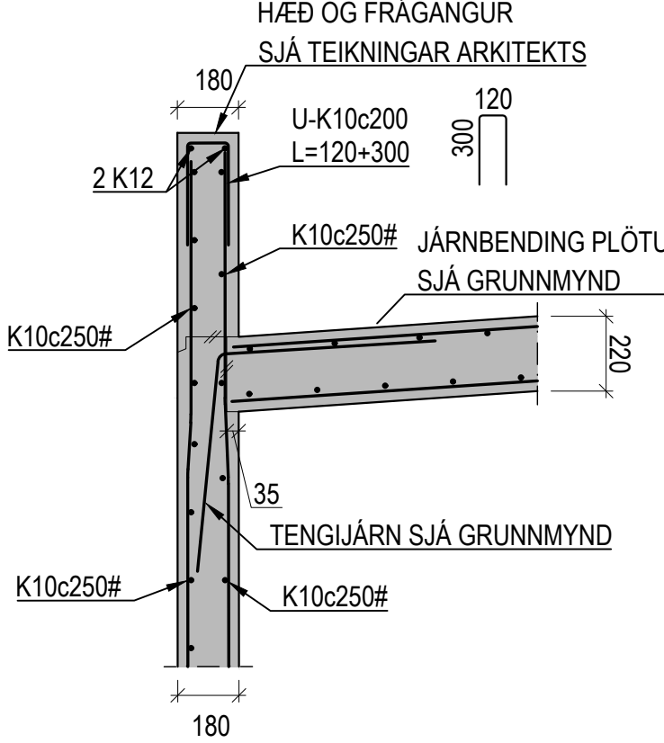
DÆMIGERT SNIÐ: TENING ÞAKPLÖTU VIÐ ÚTVEGGI 1:20
