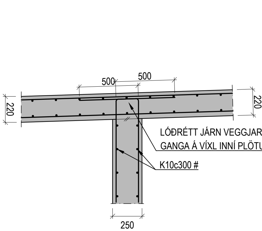
DÆMIGERT SNIÐ: TENING ÞAKPLÖTU VIÐ INNVEGGI 250 MM ÞYKKA 1:20
