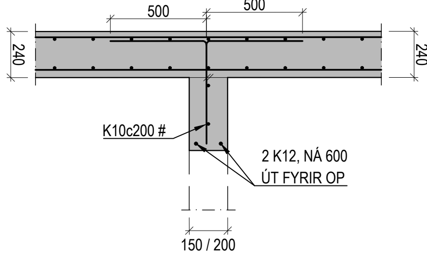
DÆMIGERT SNIÐ: TENING PLÖTU VIÐ INNVEGGI, VIÐ INNIHURÐIR, ÞAR SEM EKKI ER VEGGUR FYRIR OFAN PLÖTU 1:20
