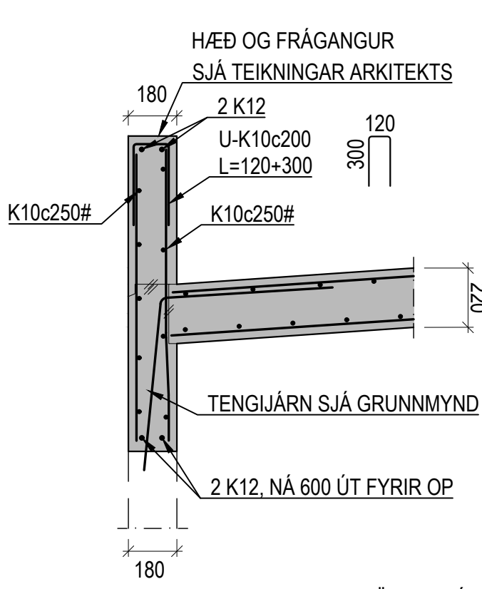
DÆMIGERT SNIÐ: TENING ÞAKPLÖTU VIÐ ÚTVEGGI ÞAR SEM GLUGGAR ERU FYRIR NEÐAN PLÖTU 1:20
